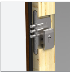
Zamek dodatkowy ryglowy
